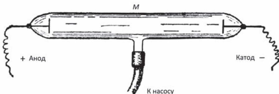
Рис. 1. Газоразрядная трубка
